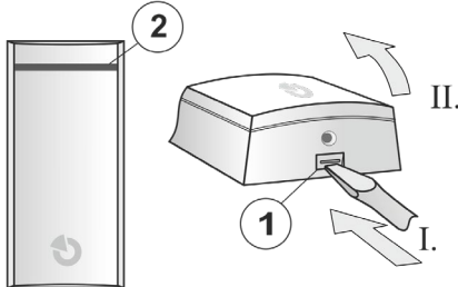
Abbildung 1: 1 – Abdeckungslasche; 2 – LED-Anzeige
