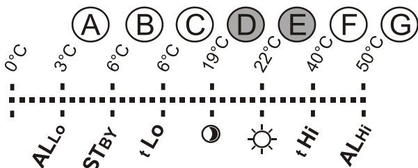
Abbeelding 2: A – Lage temperatuur, B – Temperatuur in de Standby-modus, C – Lagere temperatuurlimiet vooraf instelbaar door de gebruiker, D – Economische temperatuur, E – Comfort temperatuur, F – Hogere temperatuurlimiet vooraf instelbaar door de gebruiker, G – Hoge temperatuur
