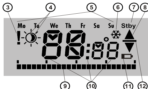
Abbeelding 3: 3 – Interne instellingen van de invoer vanuit een fout van de SW/communicatie van de F-Link; 4 – Symbolen voor de comfort* en economische temperaturen; 5 Dagen van de week 6 – verwarming geactiveerd, als de thermostaat wordt geblokkeerd; 7 – Standby-modus geactiveerd; 8 – Verwarming, knippert ▲ – thermostaat geblokkeerd door bijvoorbeeld een open raam; 9 – As van de verwarmingsperiodes; 10 – Symbolen voor het tonen van de temperatuur, tijd en tekst; 11 – Lage batterijindicator; 12 – Weergave van de vooraf ingestelde / gewenste temperatuur
