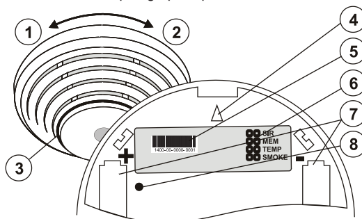
Fig. 6: 1 - Ouverture du capot du détecteur; 2 - Fermeture du capot du détecteur; 3 - Signalisation optique d'état; 4 - Flèche d'orientation pour le montage du détecteur; 5 - Code de production; 6 - Configuration des bornes; 7 - Supports des piles; 8 - Touche de test
