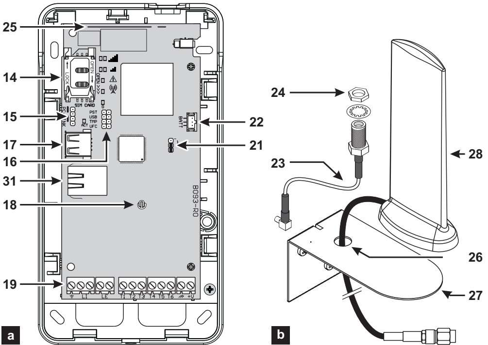
Figuur 2 – Identificatie van onderdelen: a) versie met behuizing; b) ANTLTE-02, multibandantenne met 2 m kabel en SMA-connector (optioneel).
