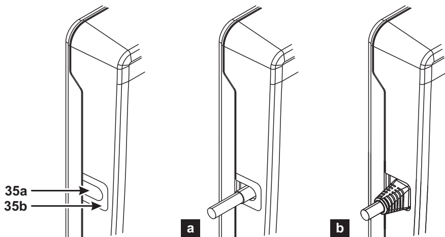
Figuur 3 – Het installeren van de communicator met behuizing.
